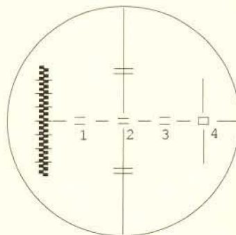
Retículo colimador modelo 381546
